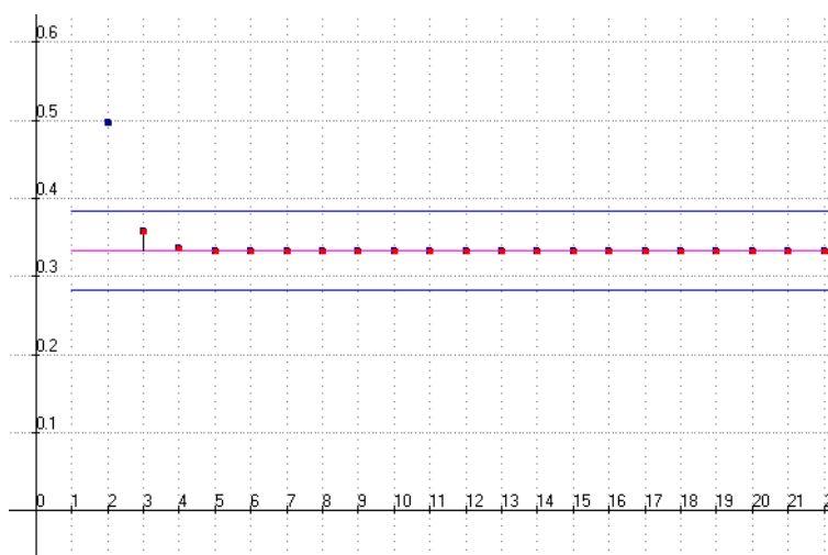
Abb.3.4.6-j: Darstellung der Folgenglieder bis n=22 , die Epsilonumgebung ist hier 0.05
