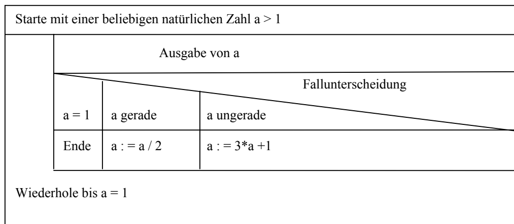
Abb. 3.4.2-a: Struktogramm zum (3a+1) -Algorithmus
