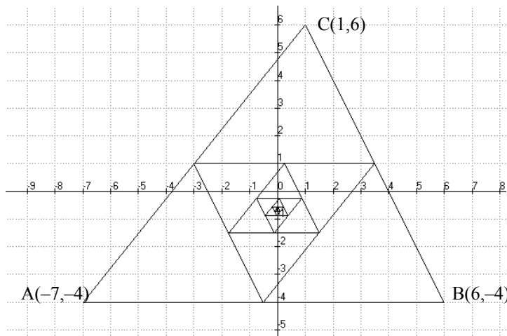
Abb.3.2-a: Seitenmittelpunkte im Dreieck, Punktfolgen A_1, A_2, A_3, \dots B_1, B_2, \dots
