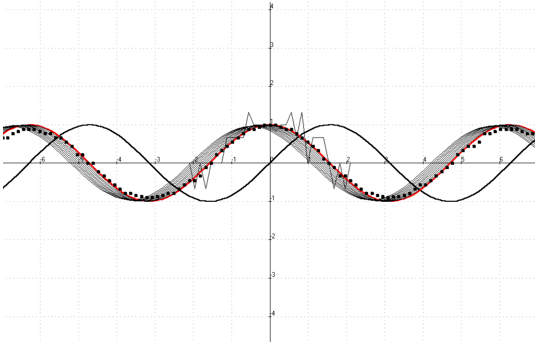
Abb. 3.4.6-h: Nun sieht auch der Punktegraph schon etwas seltsam aus! Jetzt wird u = 10^{-16} gewählt.
